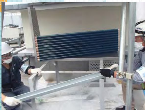
現地施工風景
