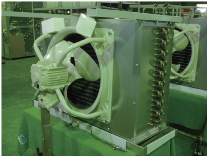
局所冷却空調機
