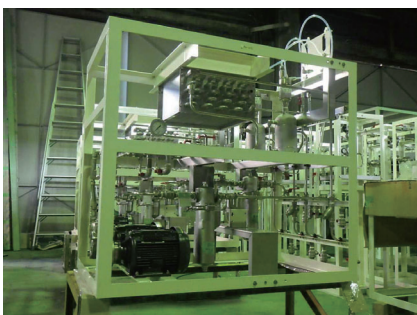
油脂類供給配管ユニット
